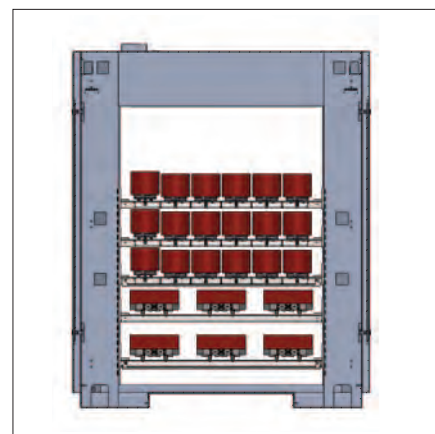
Flexible Aufteilung für unterschiedliche Palettentypen
