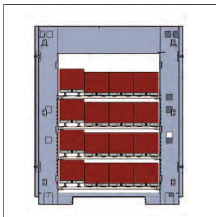
24 Palettenplätze für Palettengröße 320 x 320 mm
